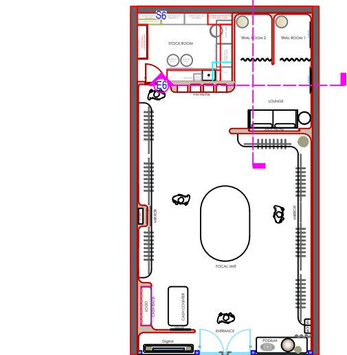
1 KEY PLAN Scale: NTS
