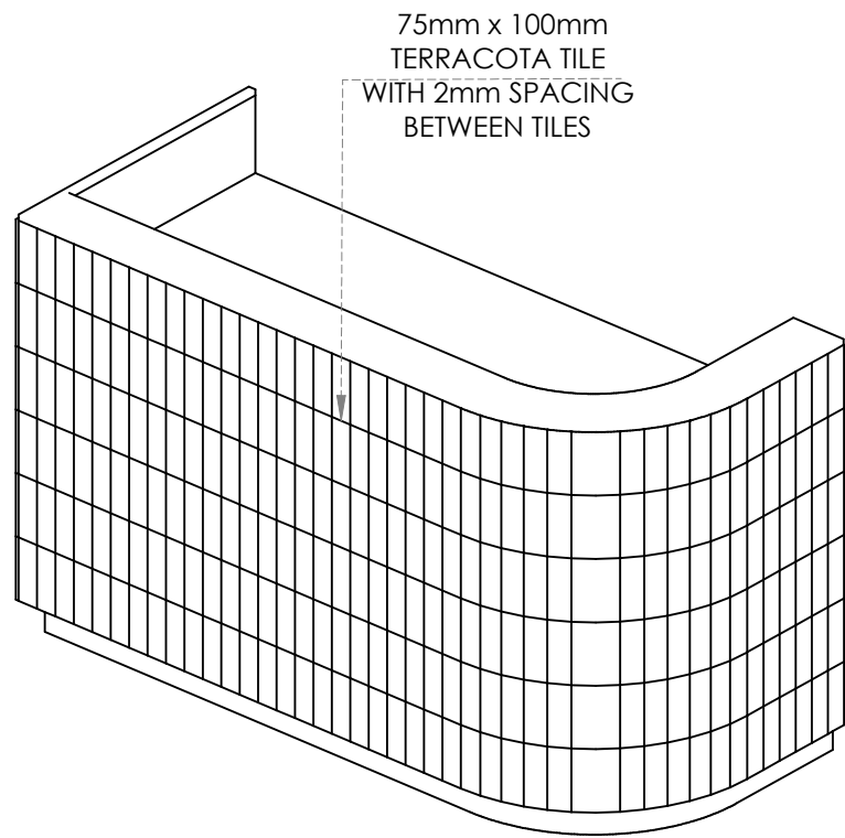
ISO - FRONT VEIW
