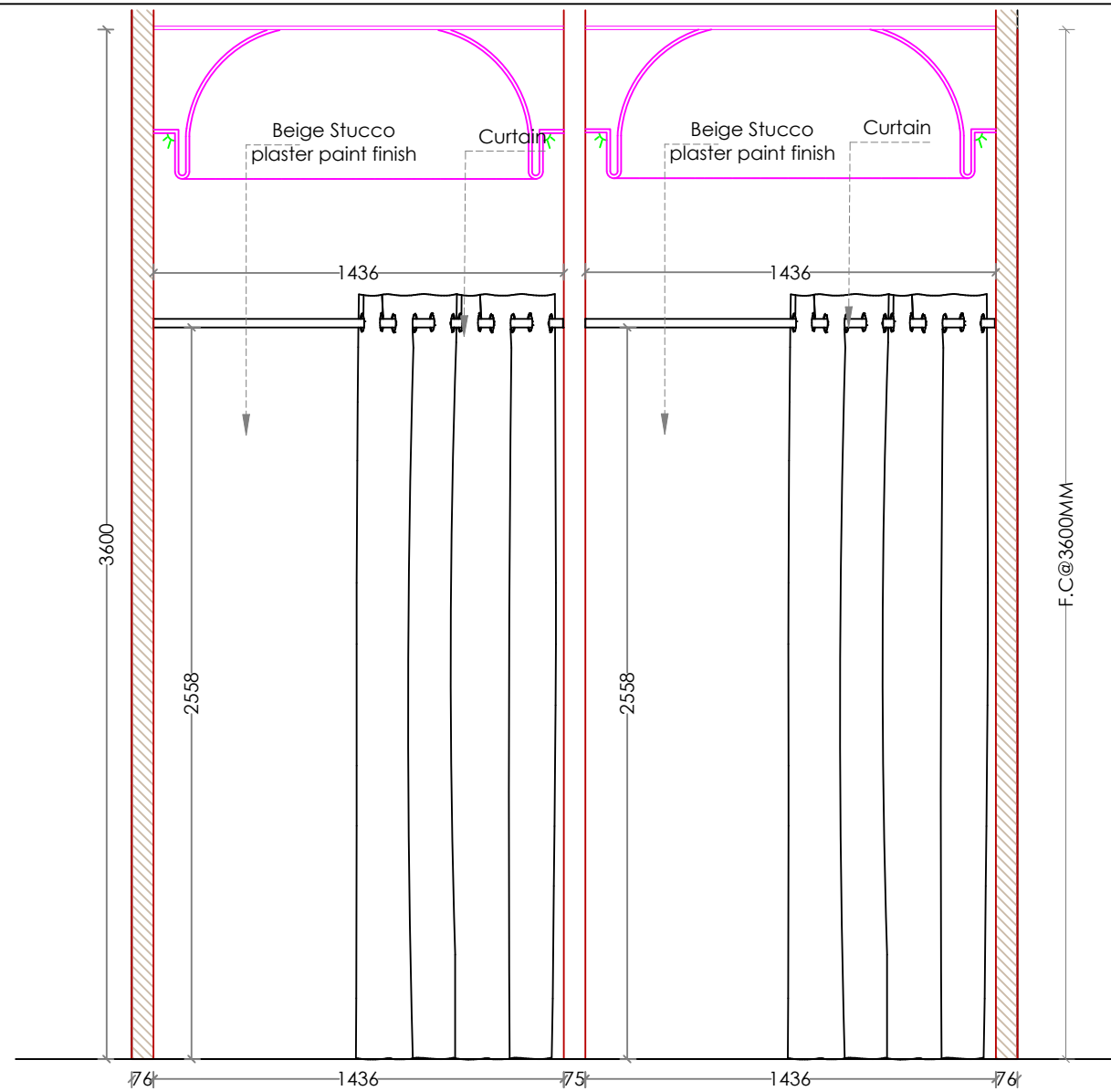
8 ELEVATION E8 Scale: NTS
