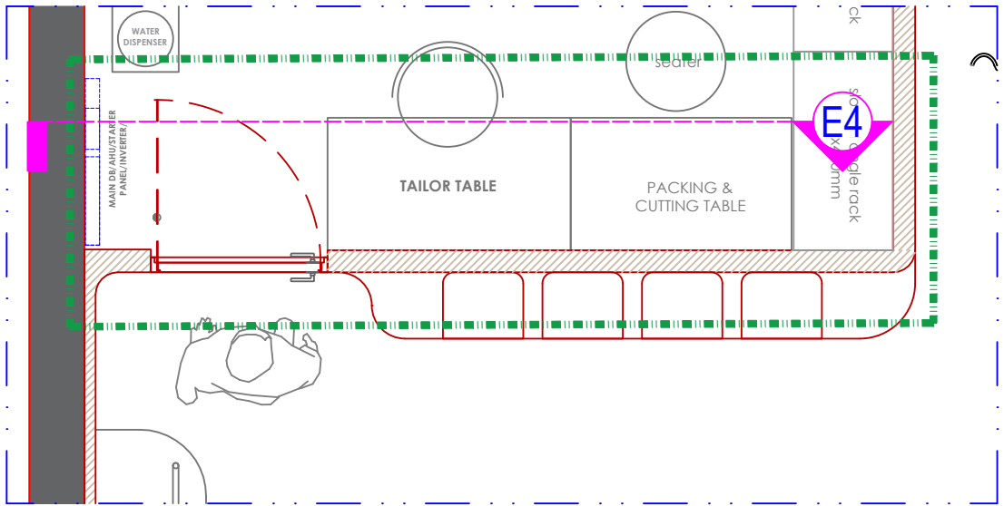
1 KEY PLAN Scale: NTS
