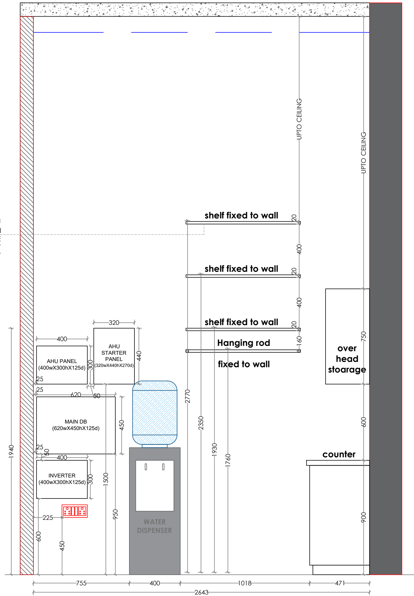
2 ELEVATION E2 Scale: NTS
