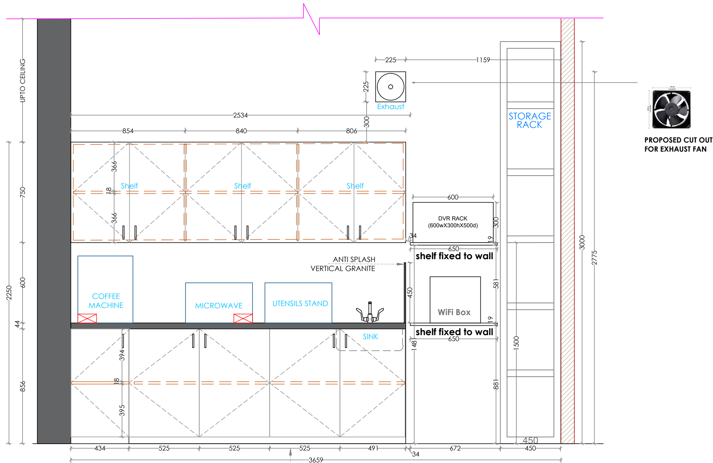
1 ELEVATION E1 Scale: NTS
