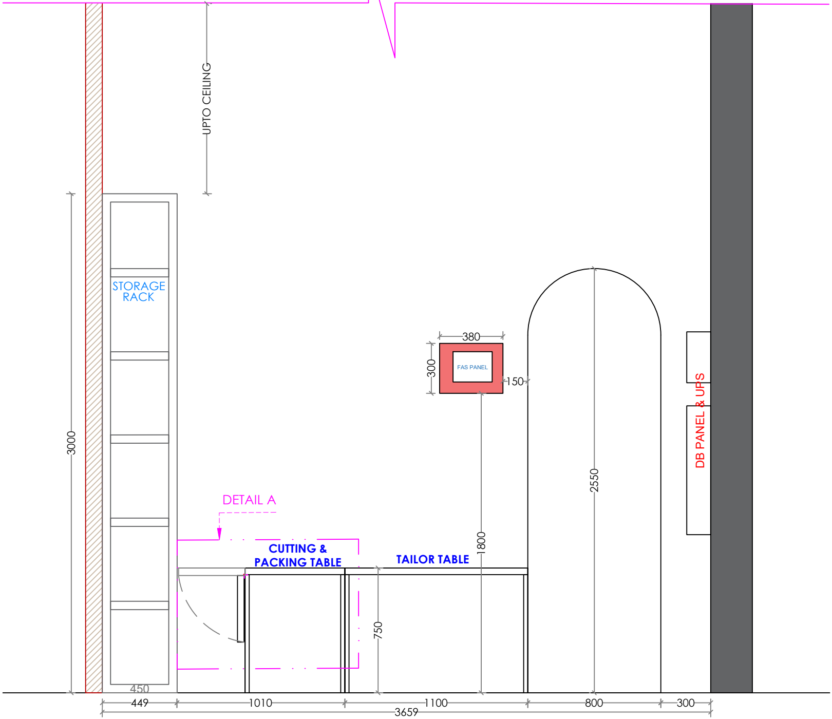
4 ELEVATION E4 Scale: NTS
