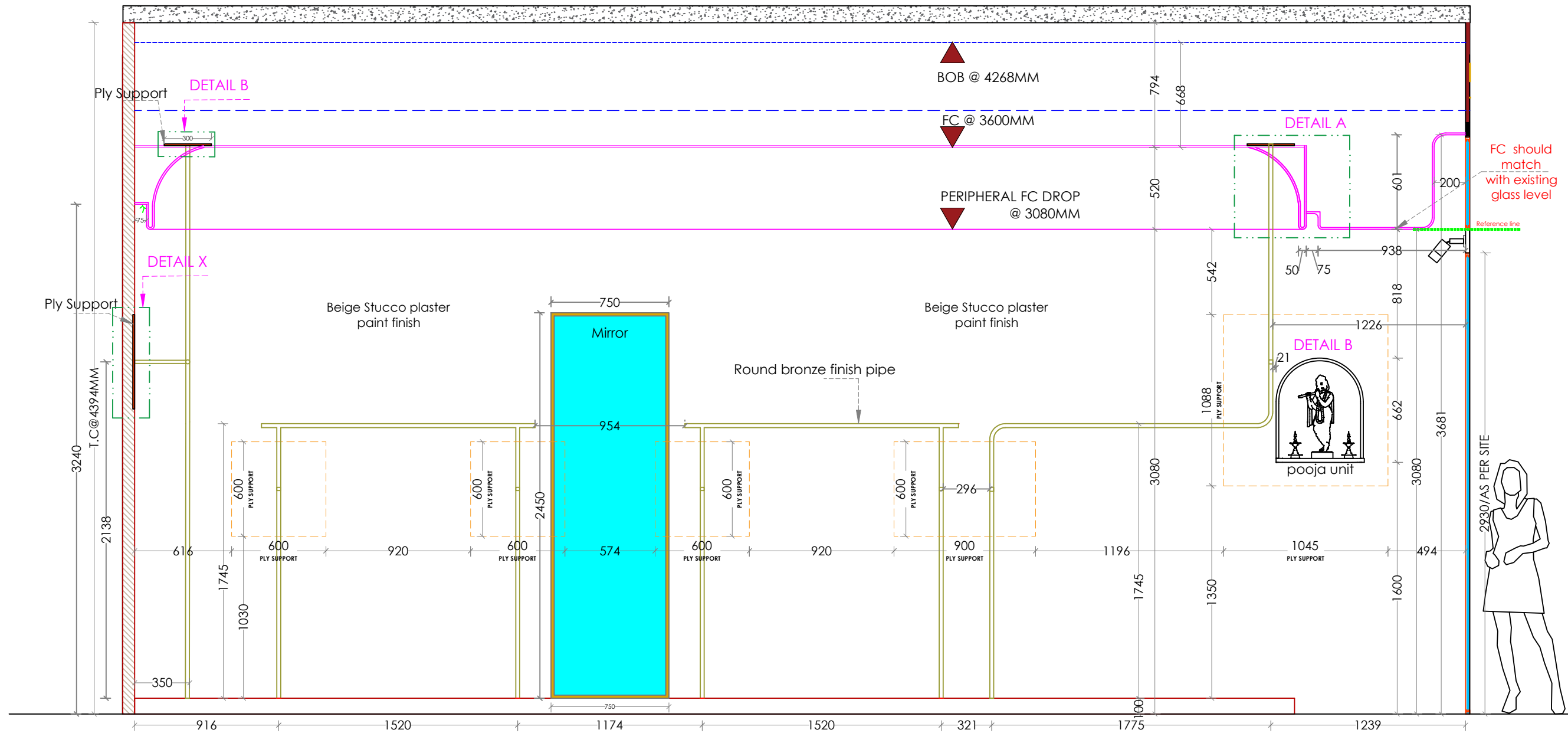
1 ELEVATION E1 Scale: NTS
